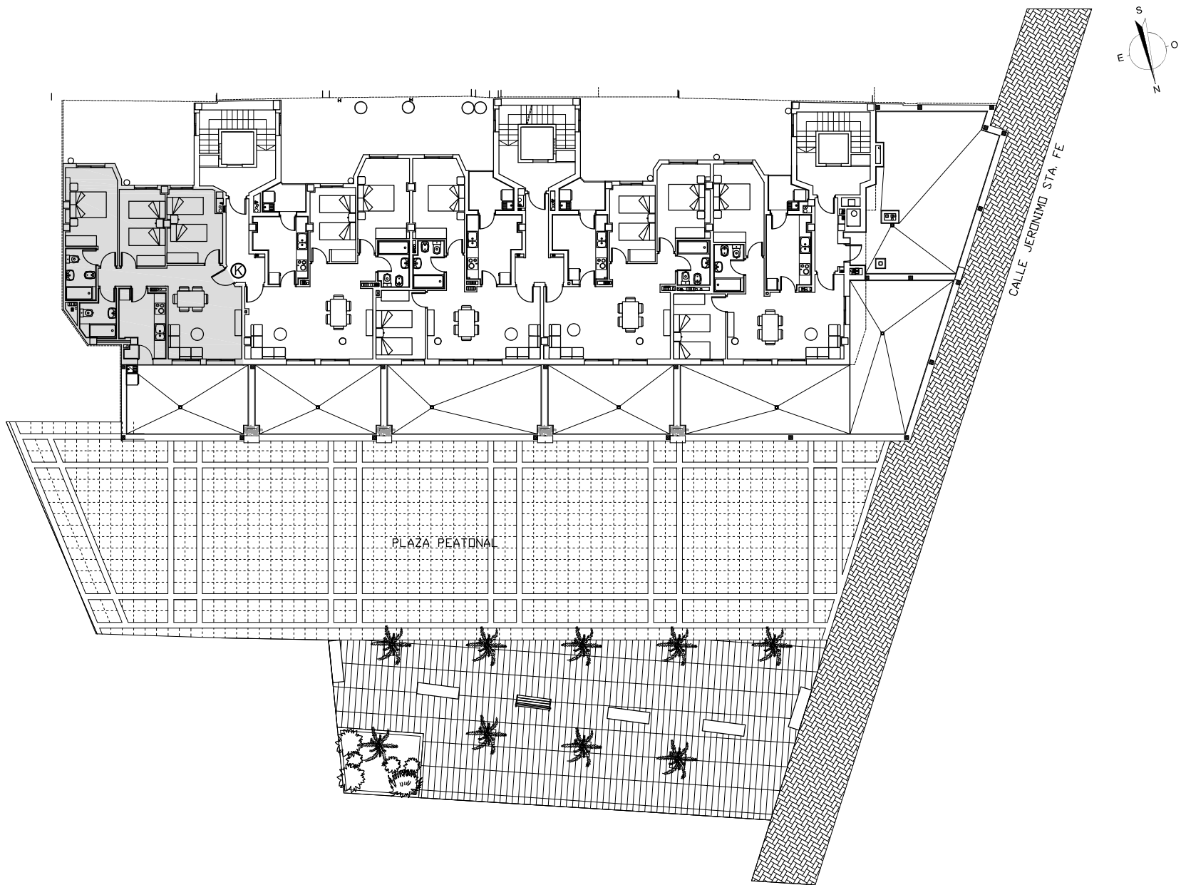
LOCALIZACION VIVIENDAS TIPO "K"
