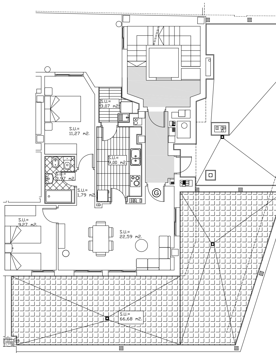
VIVIENDA TIPO "G" EN PLANTA ATICO: ESCALERA 1
