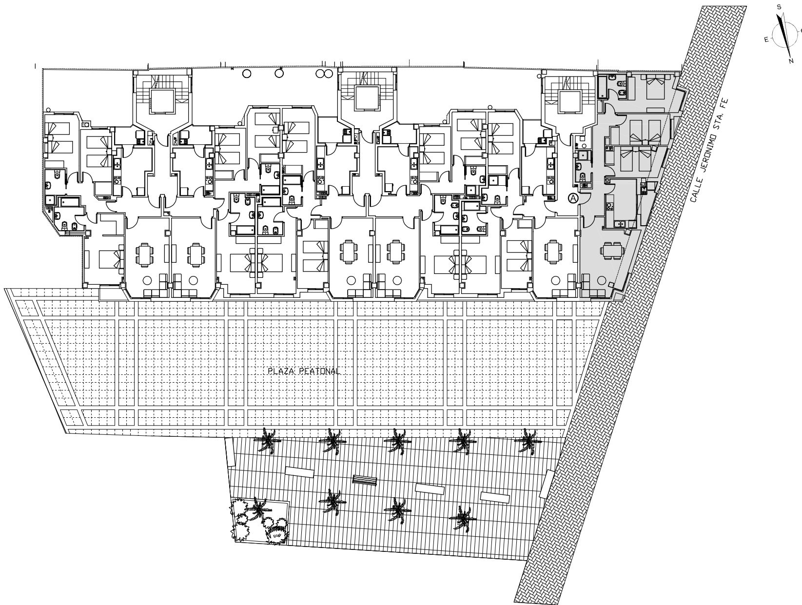
LOCALIZACION VIVIENDAS TIPO "A"
