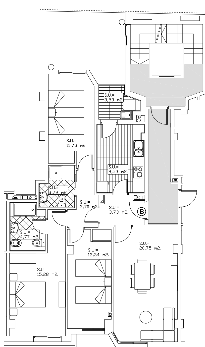
VIVIENDA TIPO "B" EN PLANTA SEGUNDA; ESCALERA 1
